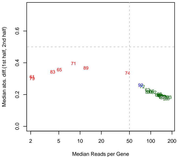
6/11/2014 pseudo3_N2E3_ML2_set2 mad12
