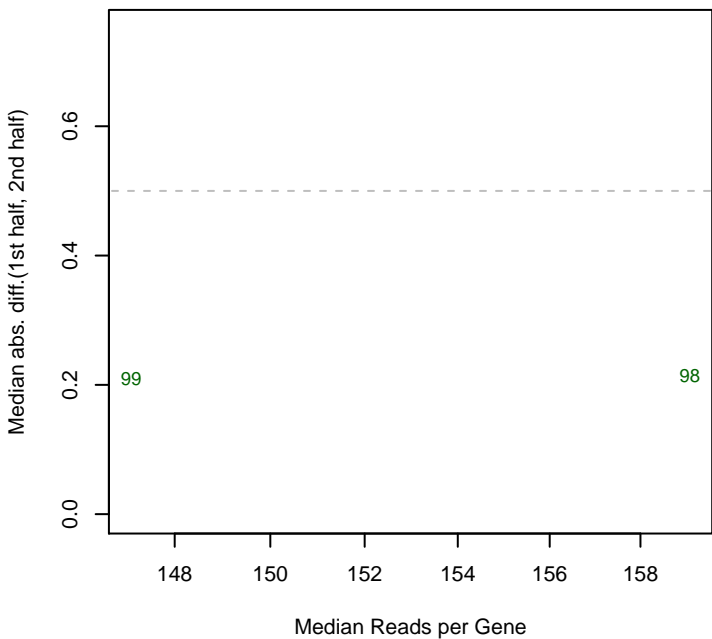
6/11/2014 pseudo3_N2E3_ML2_set3 mad12
