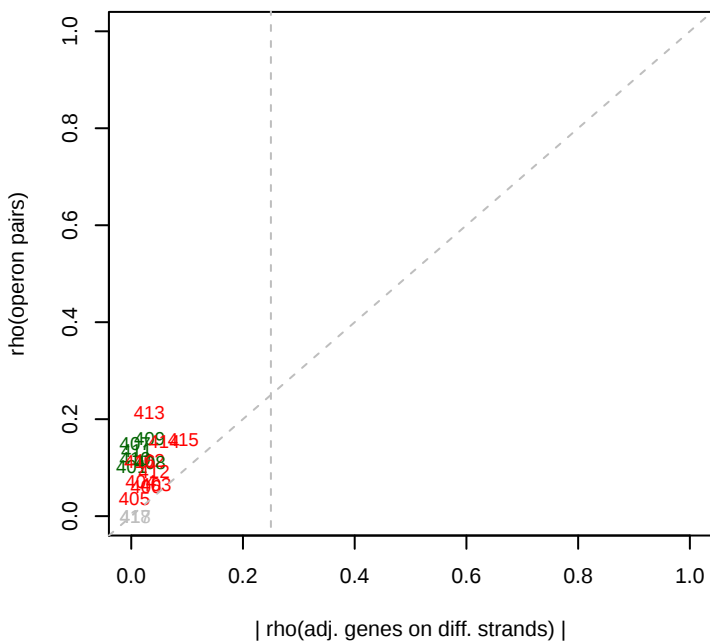
1/26/2015 Phaeo_ML1_set9 rho(opérons)
