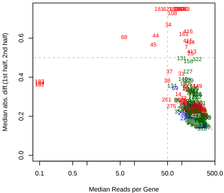
Phaeo mad12
