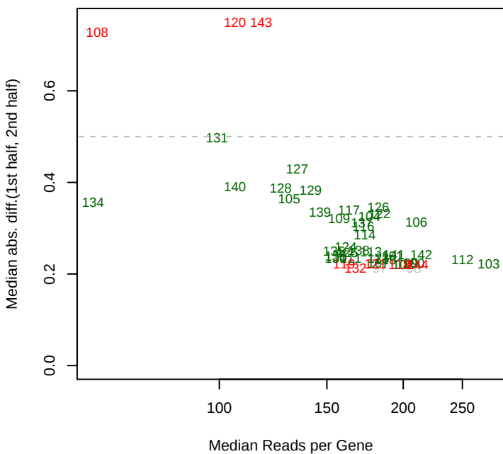
8/5/2013 Phaeo_ML1_set3 mad12
