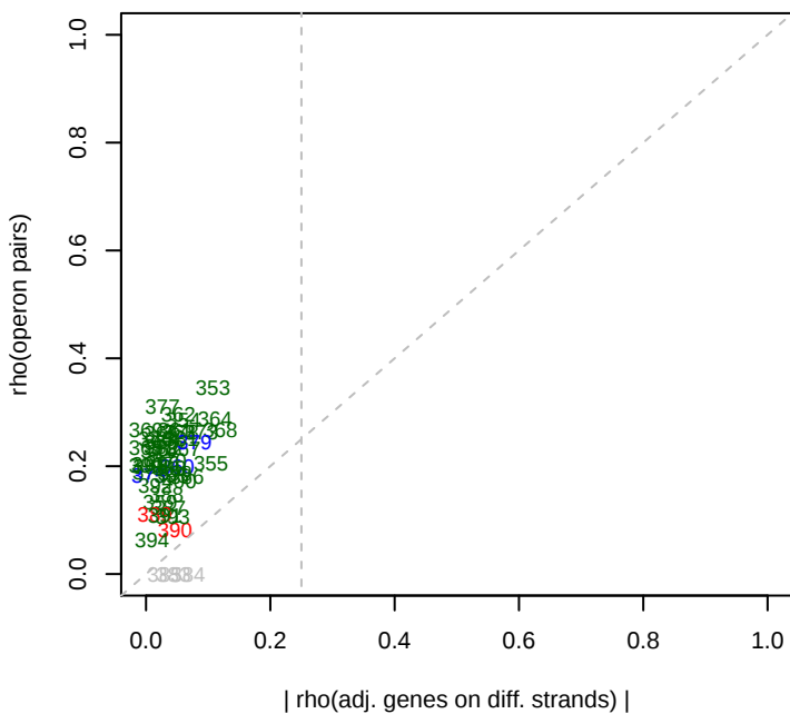
1/20/2015 Phaeo_ML1_set8 rho(opérons)
