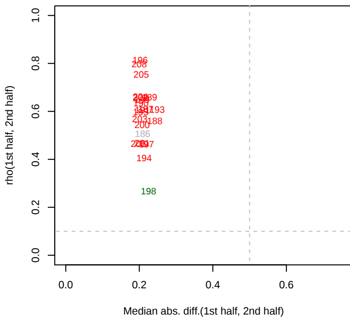
10/23/2013 Phaeo_Dino_combined_set rho12
