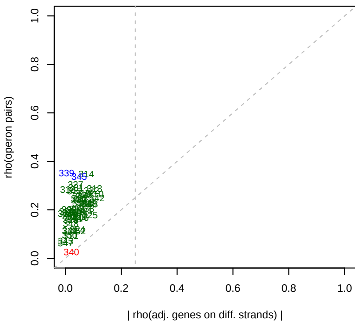
marchapr14 rho(opérons)
