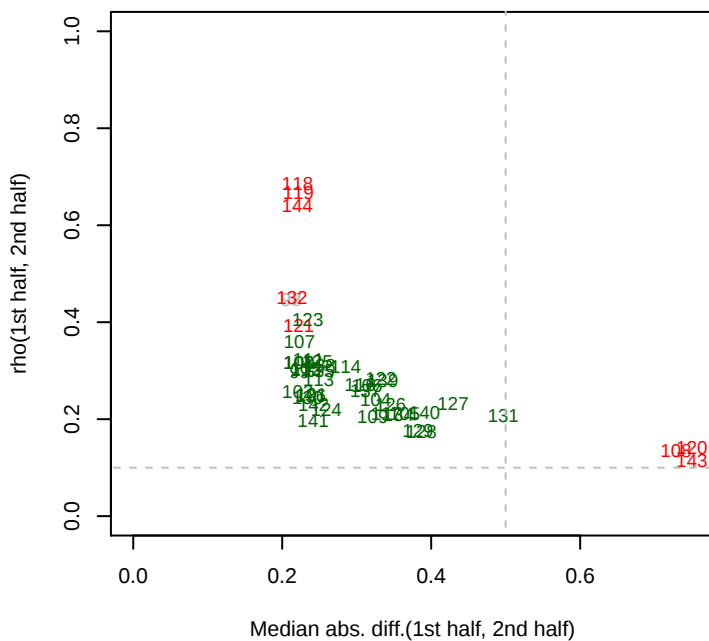
8/5/2013 Phaeo_ML1_set3 rho12
