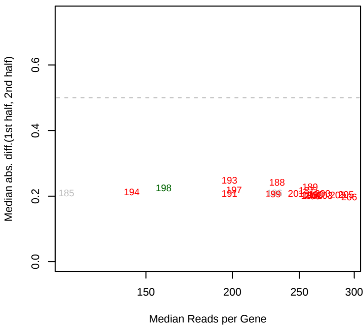
10/23/2013 Phaeo_Dino_combined_set mad12
