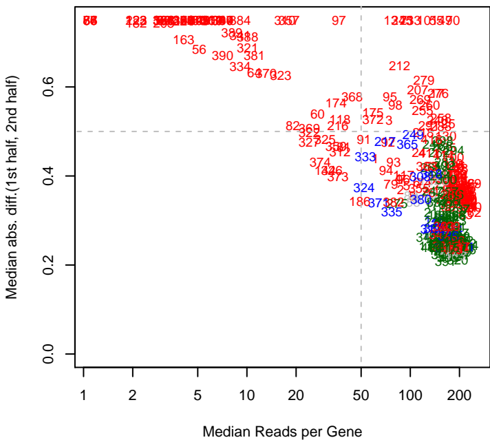
Koxy mad12
