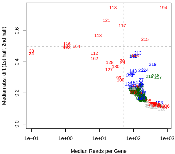
Keio mad12
