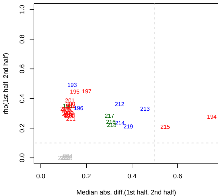
2/2/2015 Keio_ML9_set6 rho12
