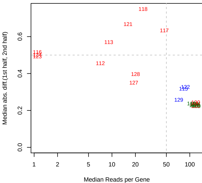
6/24/2014 Keio_ML9_set2 mad12
