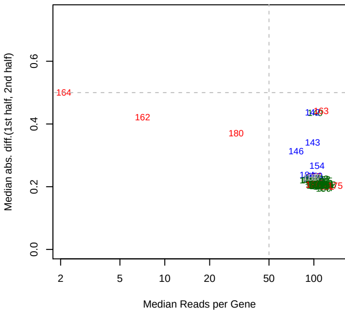
6/30/2014 Keio_ML9_set2 mad12
