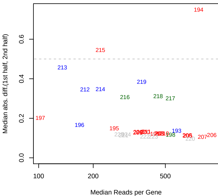
2/2/2015 Keio_ML9_set6 mad12
