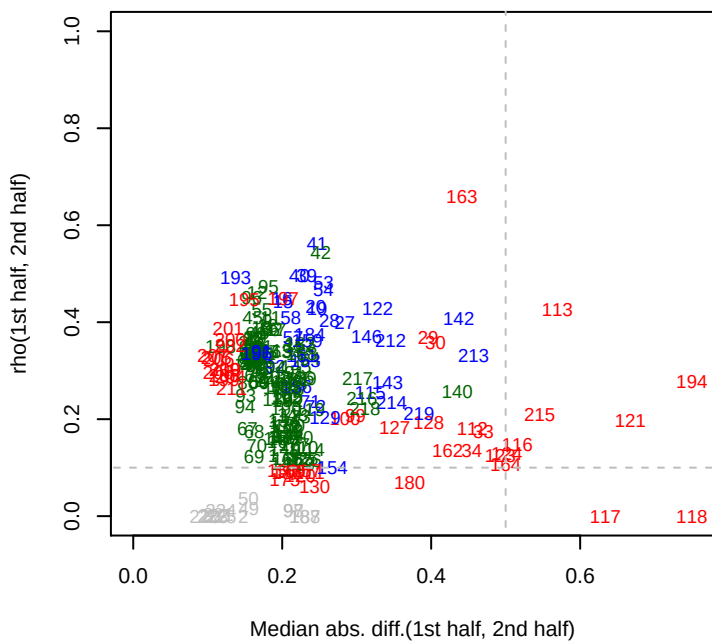
Keio rho12
