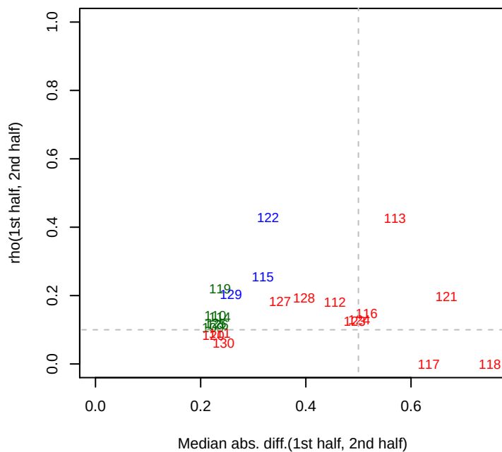
6/24/2014 Keio_ML9_set2 rho12
