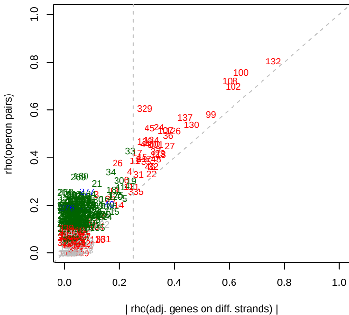
Dino rho(opérons)
