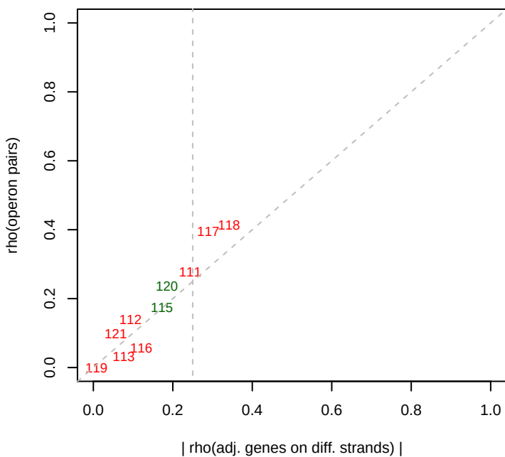
8/22/2013 rho(opérons)
