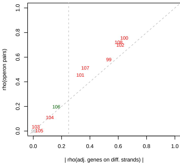
6/6/2013 Marino_Dino_extra_set rho(operons)
