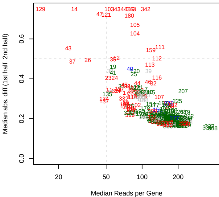
Dino mad12
