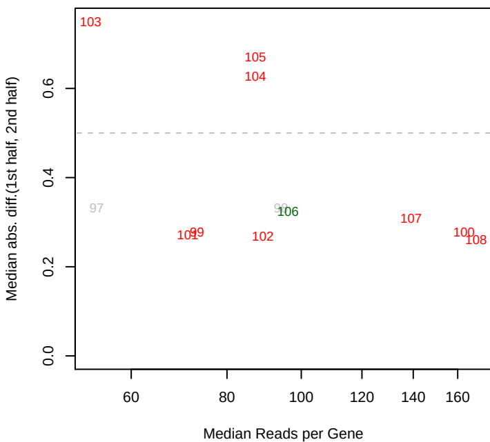
6/6/2013 Marino_Dino_extra_set mad12
