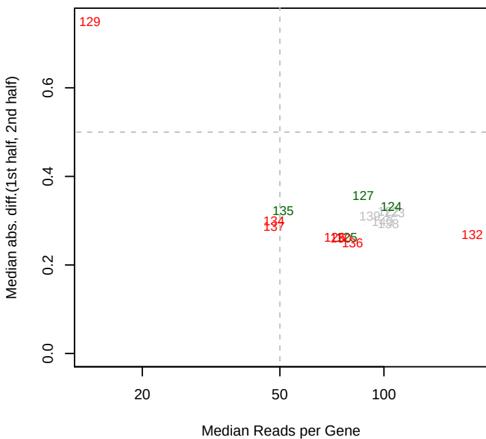
10/23/2013 Phaeo_Dino_combined_set mad12
