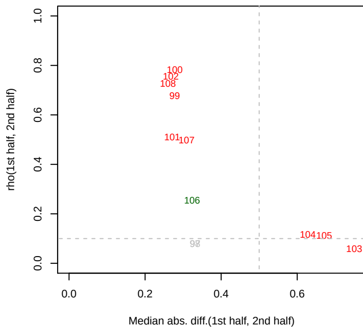
6/6/2013 Marino_Dino_extra_set rho12
