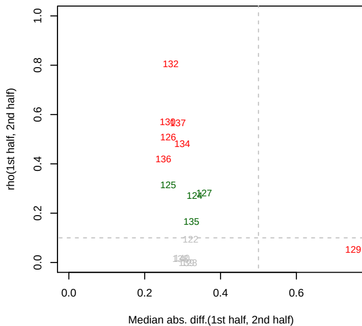
10/23/2013 Phaeo_Dino_combined_set rho12
